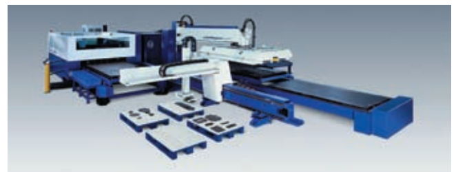
LiftMaster und SortMaster für die Zu- und Abführung von Rohblechen bei Flachbettlaser-Schneideanlagen
