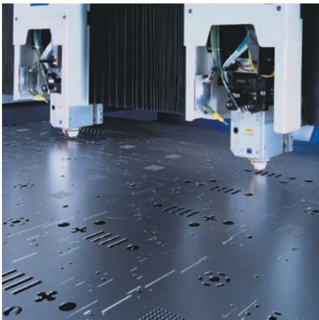
Hochgeschwindigkeits-Laser-Schneidemaschine Trumatic HSL 2502
