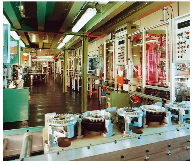
Automatische Fertigungslinie für Visco®-Lüfterkupplungen.
