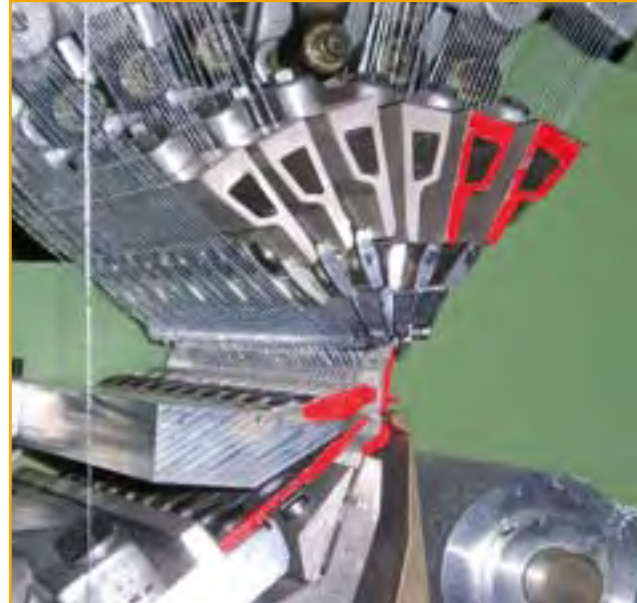
Wirkelemente einer Laborwirkmaschine
