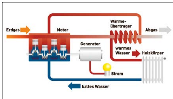
Prinzip des BHKW
