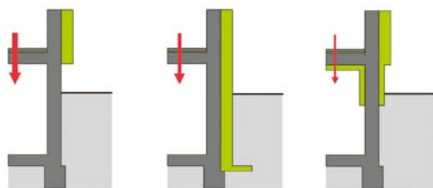
Dämmvarianten der Hausfassade
