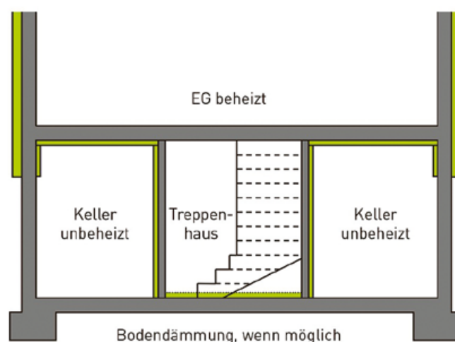
Querschnitt
