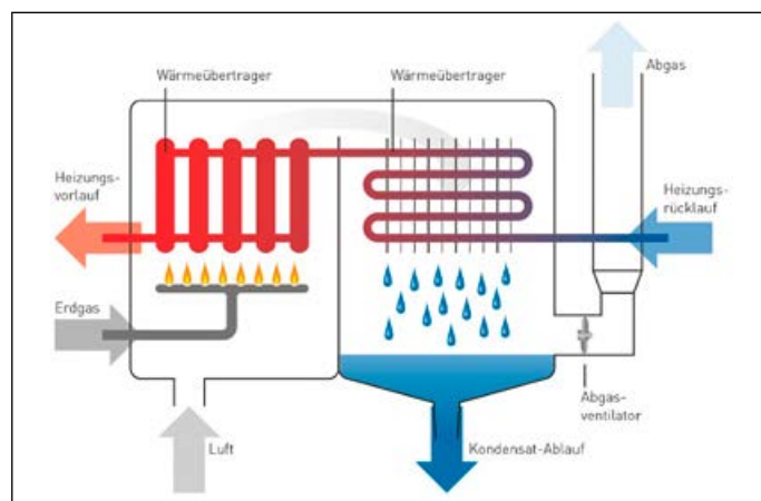
Prinzip des Gasbrennwertkessels
